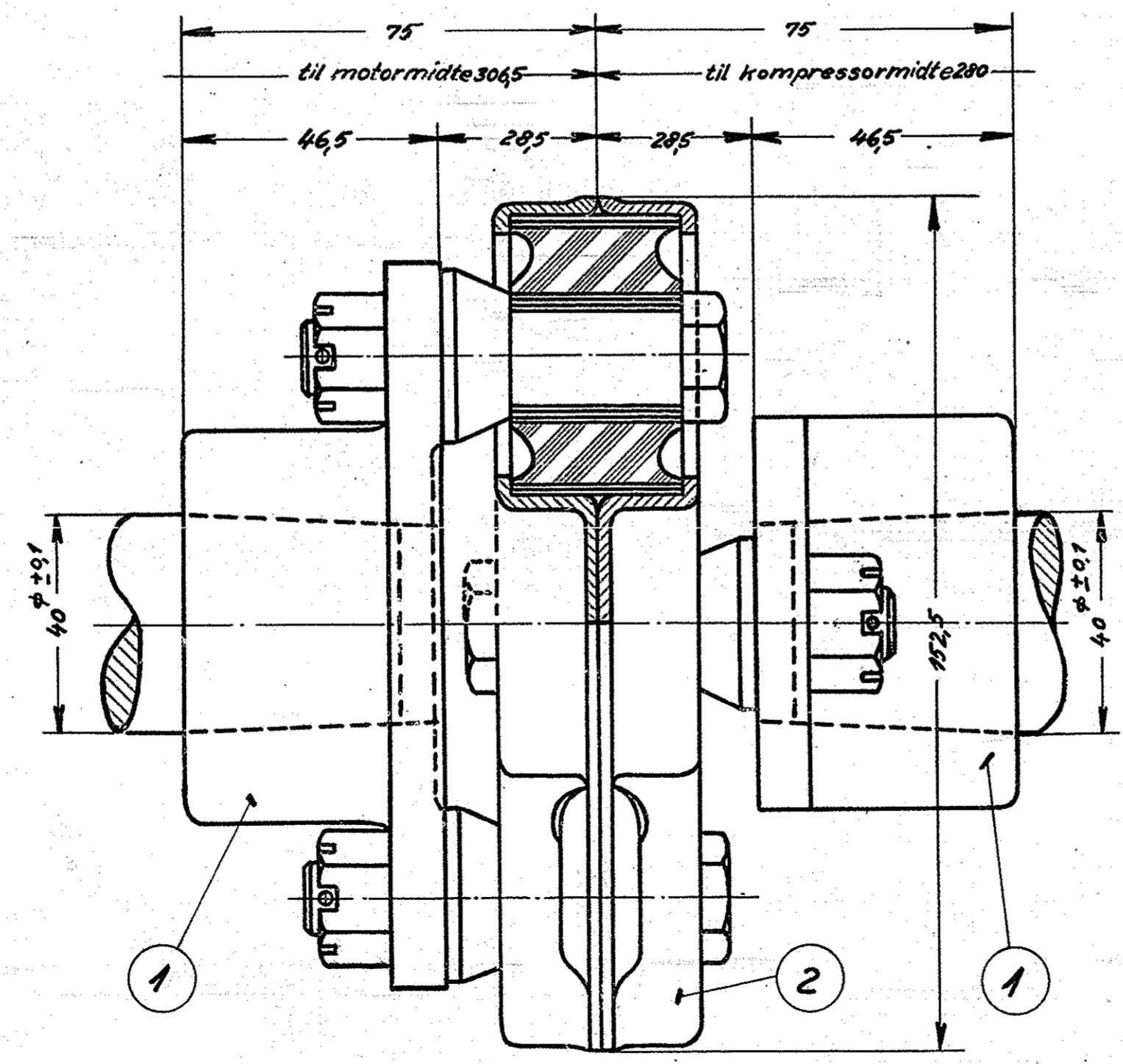
LAYRUP kobling nr. 60 x 1 1/4 2 tegn.nr. 11432.
